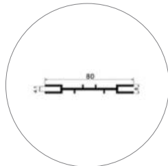
CABO-SEG-PLASTIC 82.95" W (qty 8)
