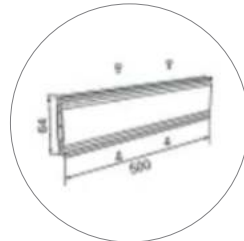
CABO-80 ADPT (qty 27)
